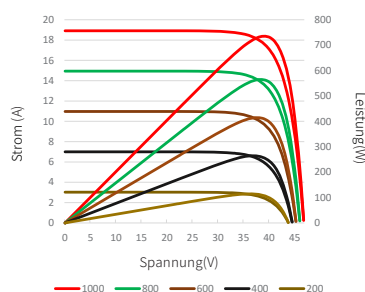
Strom-Spannungs- und Leistungs-Spannungs-Diagramme(700W)
